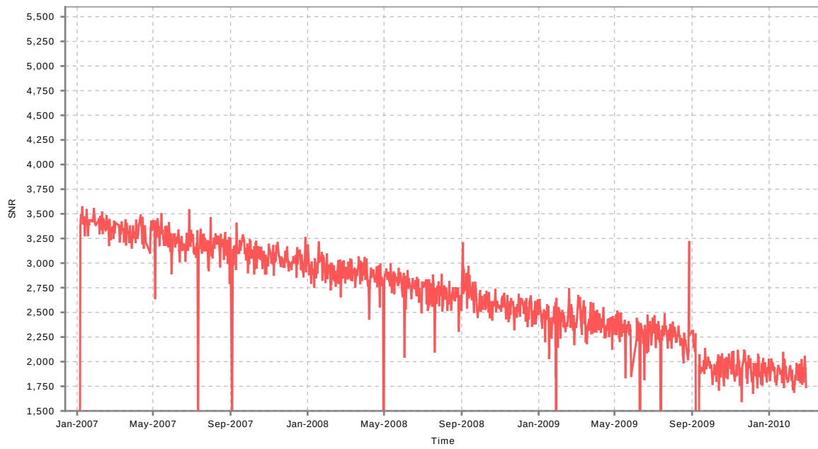
SNR (WLS) @310nm
